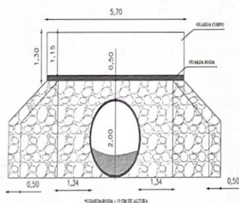
4 VISTA FRONTAL Escala 1:50
