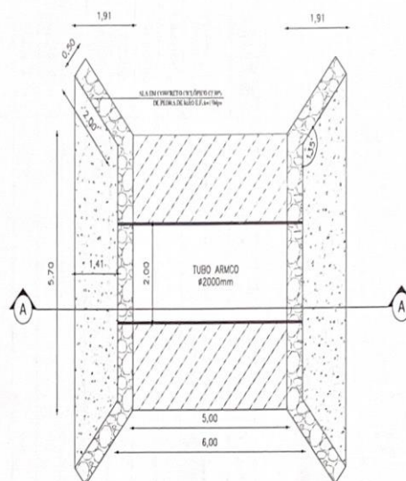
2 PLANTA BAIXA Escala 1:10
