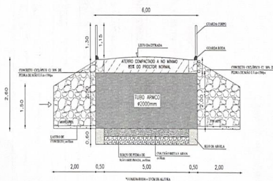
5 CORTE AA Escala 1:50
